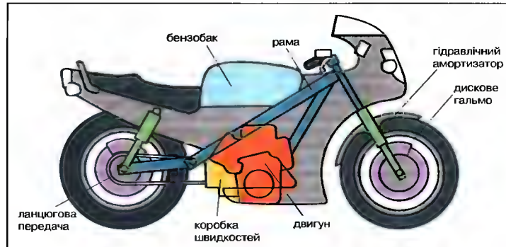
Спортивний мотоцикл Головні частини мотоцикла
